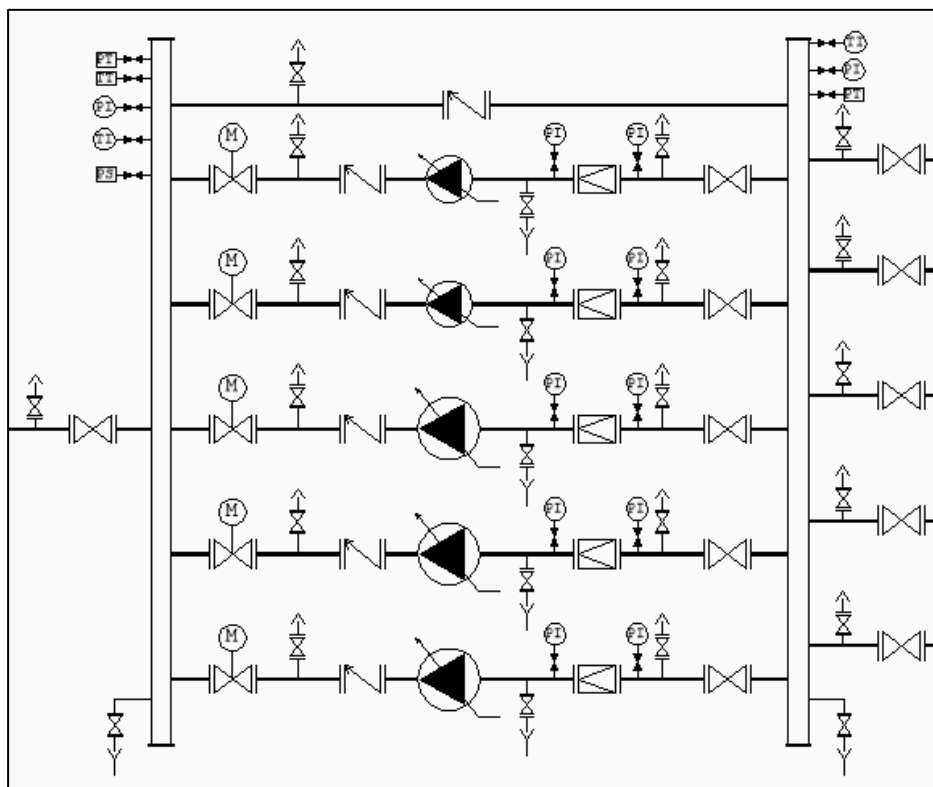
Εικόνα 4: Ελάχιστες απαιτήσεις εξοπλισμού και ενδεικτική συνδεσμολογία σωληνογραμμών αντλιών του αντλιοστασίου κυκλοφορίας συστήματος μεταφοράς
