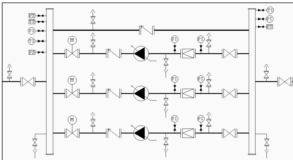
Εικόνα 3: Ελάχιστες απαιτήσεις εξοπλισμού και ενδεικτική συνδεσμολογία σωληνογραμμών αντλιών του αντλιοστασίου κυκλοφορίας συστήματος παραγωγής
