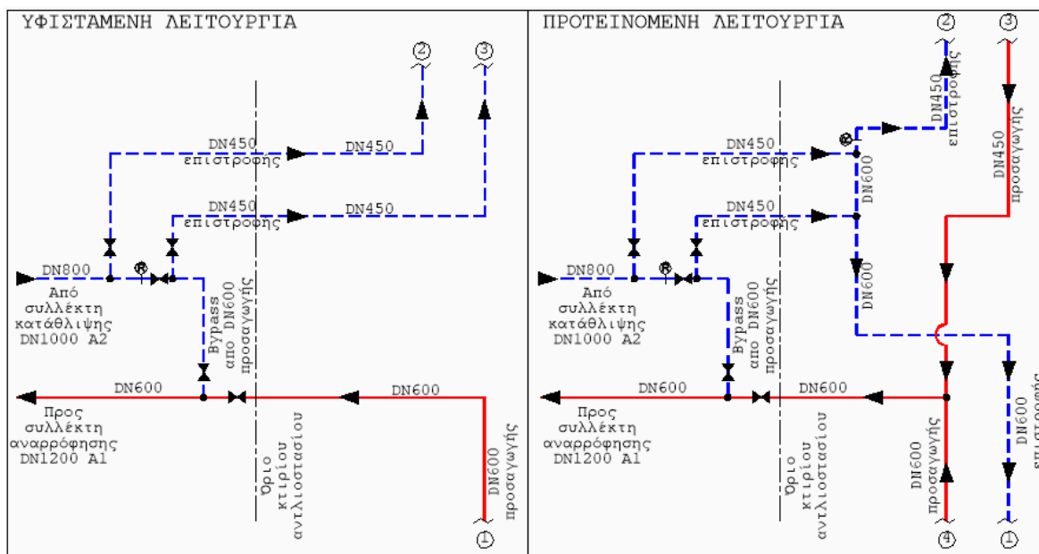
Εικόνα 5: Υφιστάμενη και προτεινόμενη συνδεσμολογία αγωγών μεταφοράς
