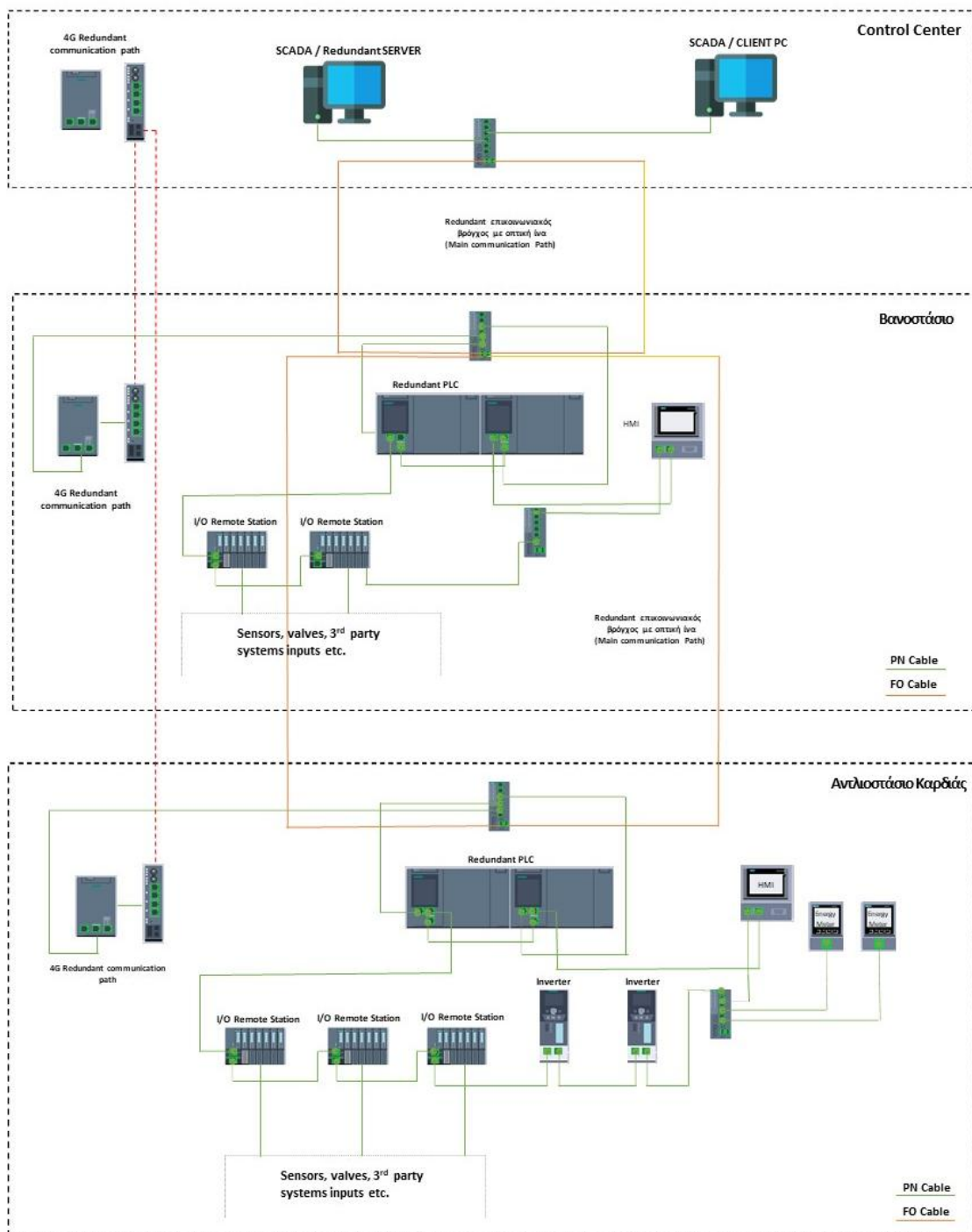
Εικόνα 6: Σχηματική διάταξη αυτοματισμού
