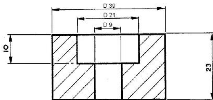
Κυλινδρικό πόδι ηλεκτροδίου Τομή Α- Α
