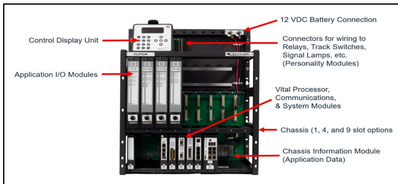
Εικόνα: ElectroLogIXS VLC 9-slot
