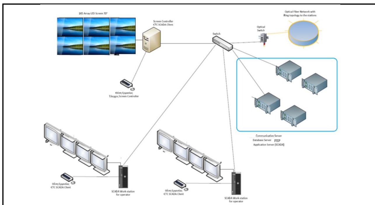
Εικόνα: Αρχιτεκτονική συστήματος TMS Λάρισα
