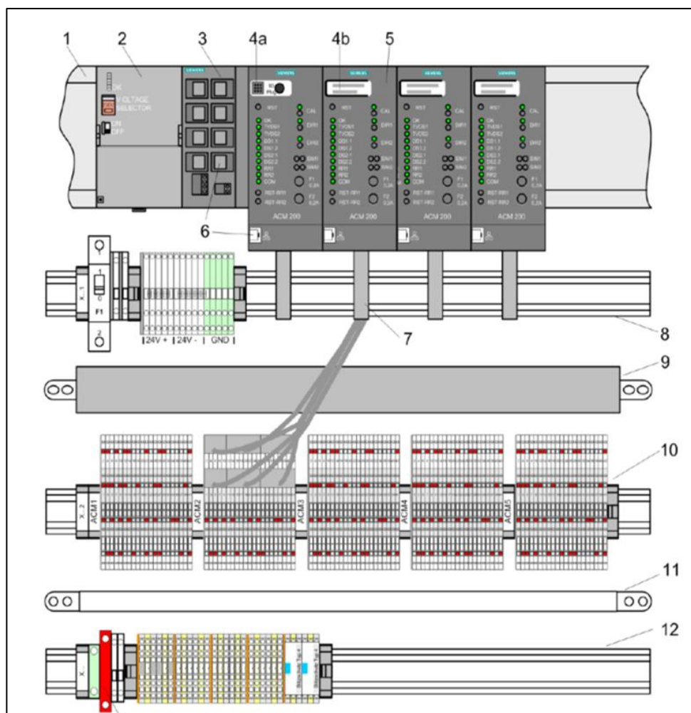
Εικόνα: Τυπική εσωτερική εγκατάσταση ACM 200
