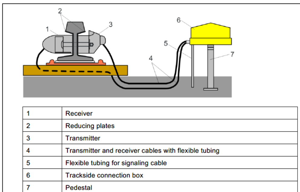
Εικόνα: Σχηματική Αναπαράσταση Παρατρόχιου Εξοπλισμού Μετρητών Αξόνων
