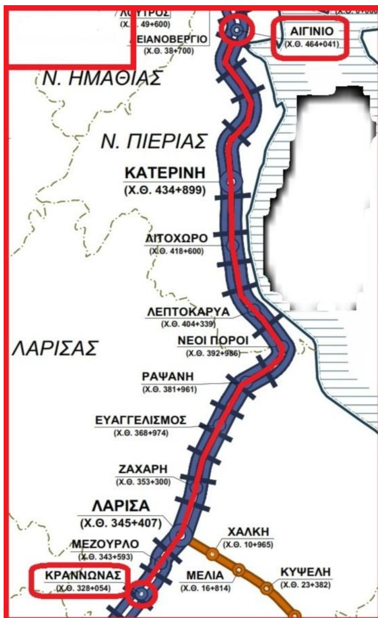
Σκαρίφημα (α): Τμήμα Σιδηροδρομικής γραμμής «Κραννώνας – Αιγίνιο»
