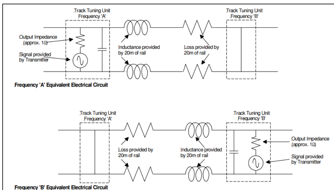
Εικόνα: Κυκλωματικά διαγράμματα περιγραφής κατευθυντικού συντονισμού
