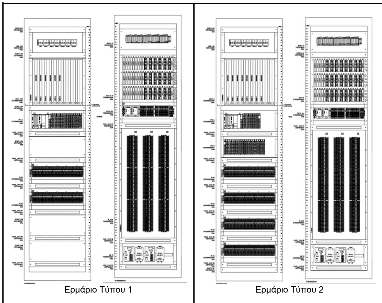
Εικόνα: Τυπικό Σχέδιο Εμπρόσθιας/ Οπίσθιας Όψης ερμαρίων Τύπου 1 & Τύπου 2 PLC X20 B&R
