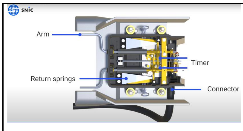
Εικόνα: Σχηματική Αναπαράσταση Μηχανικής Τροχοεπαφής Forfex (A-B) 086/046310
