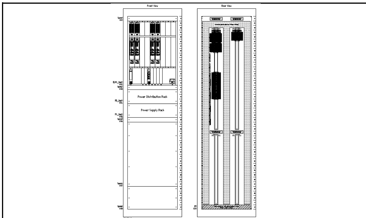
Εικόνα: Τυπικό Σχέδιο Εμπρόσθιας/ Οπίσθιας Όψης ερμαρίου ElectroLogIXS
