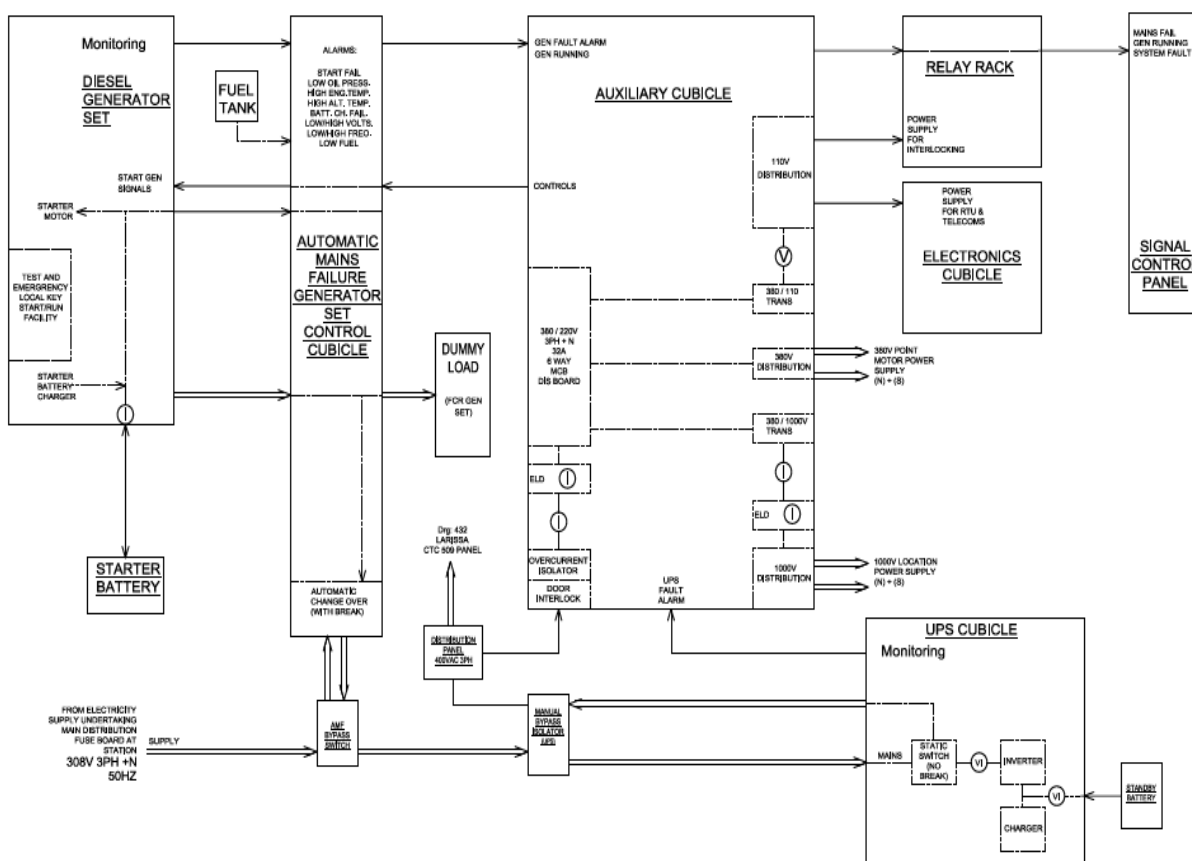
Εικόνα: Ενδεικτική Διαγραμματική απεικόνιση συστήματος τροφοδοσίας σηματοδότησης-τηλεδιοίκησης
