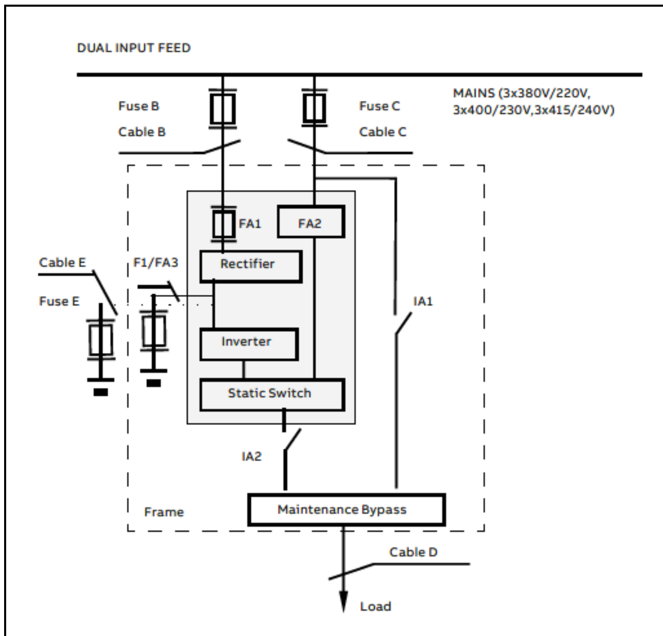
Εικόνα: Διαγραμματική απεικόνιση συστήματος αδιάλειπτης τροφοδοσίας σηματοδότησης-τηλεδιοίκησης
