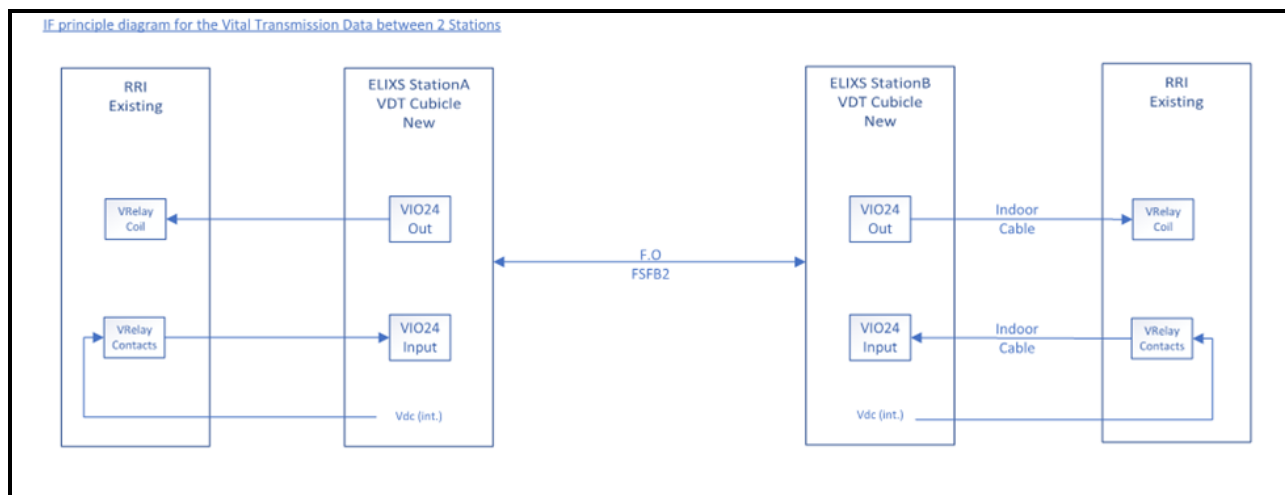
Εικόνα: Μετάδοση ζωτικών δεδομένων – ElectroLogIXS
