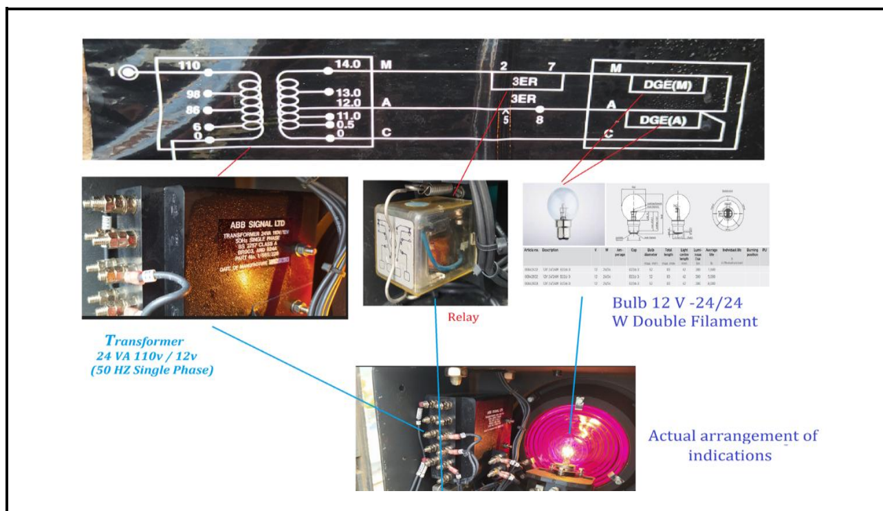
Εικόνα: Κύκλωμα ελέγχου λάμπας διπλού νήματος
