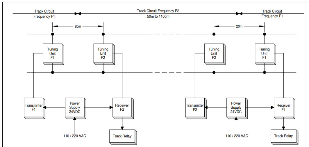
Εικόνα : Μπλοκ διάγραμμα «βασικού» κυκλώματος γραμμής
