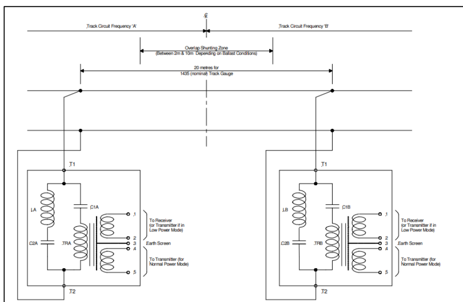
Εικόνα: Περιγραφή λειτουργίας ηλεκτρικού αρμού διαχωρισμού
