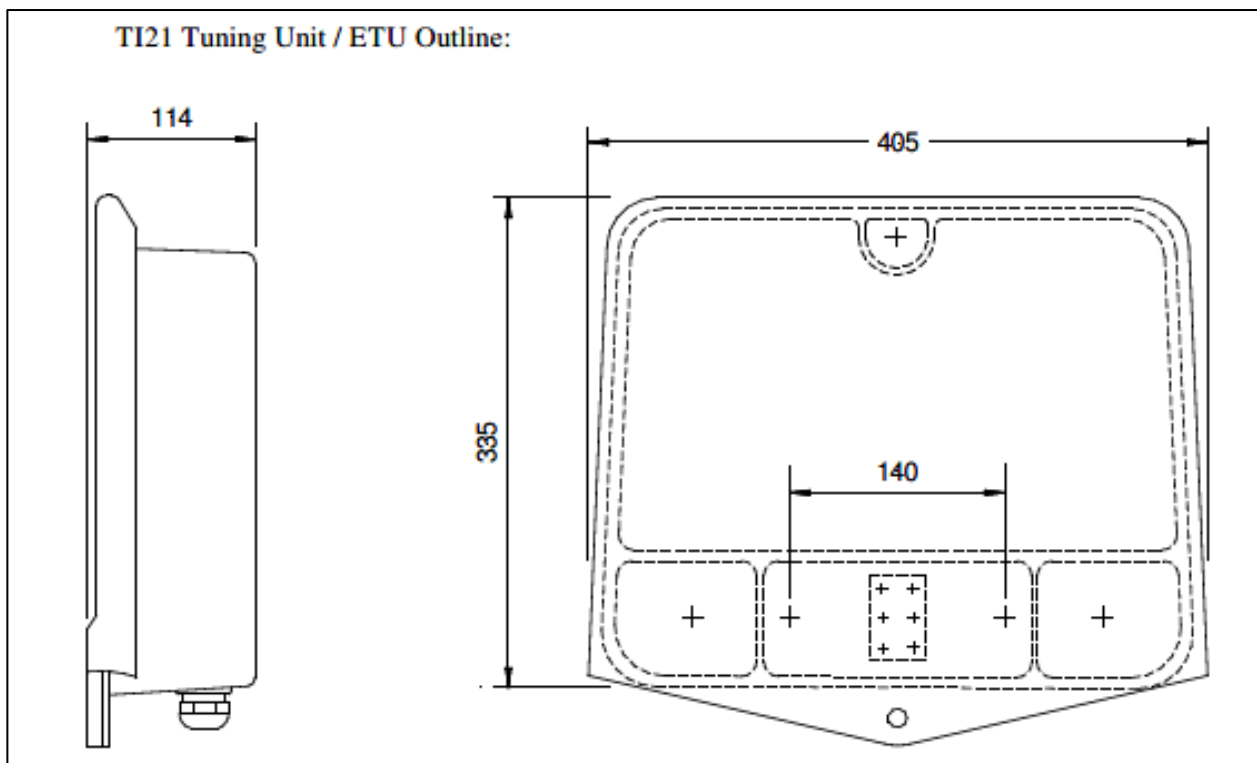
Εικόνα: Μονάδες συντονισμού- Τερματικές μονάδες συντονισμού
