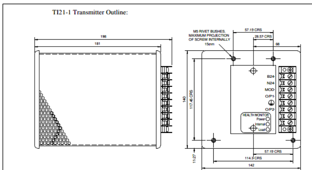
Εικόνα: Πομπός TI21
