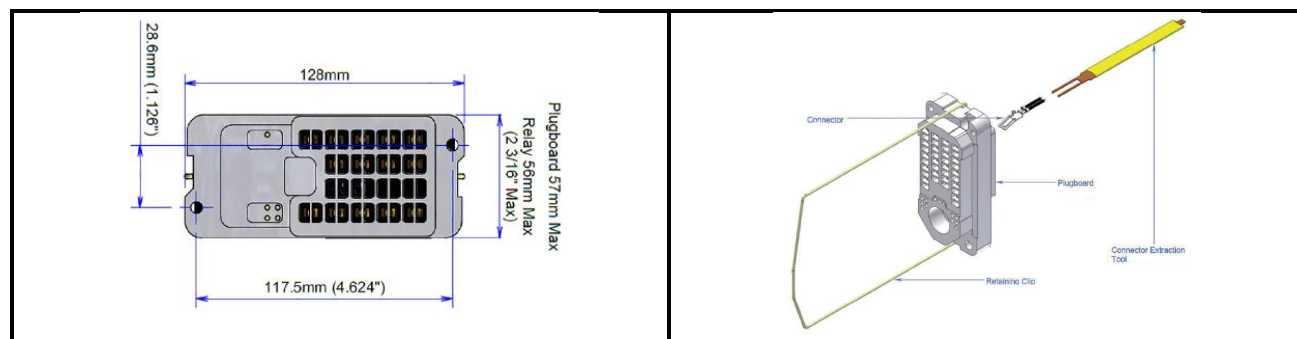
Εικόνα: Τυπικό Σχέδιο Ηλεκτρονόμου Q-Style
