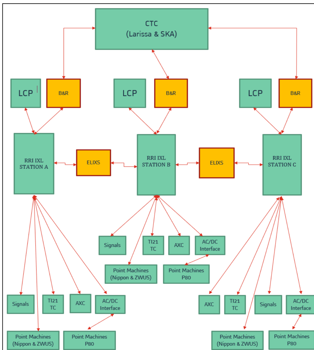
Γενική Αρχιτεκτονική Συστήματος Σηματοδότησης-τηλεδιοίκησης Τμήματος
