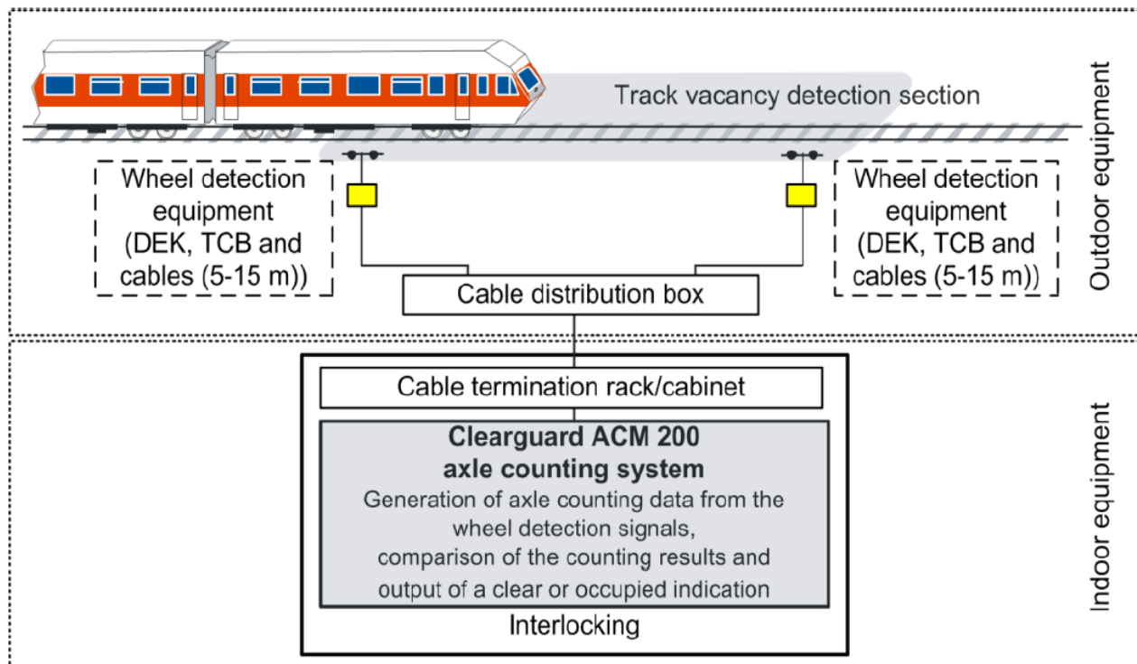
Εικόνα: Σχηματική Αναπαράσταση Συστήματος Μετρητών Αξόνων
