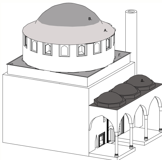
Εικ. Τα διακριτά στάδια της μολυβδοκάλυψης της εξωτερικής επιφάνειας της στέγης.
