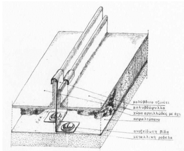
Εικ.: Κατασκευαστικές λεπτομέρειες μολύβδινης επικάλυψης
