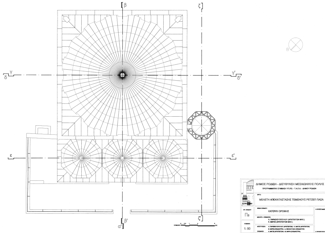
Εικ.: Κάτοψη οροφής Τεμένους Ρετζέπ Πασά.
