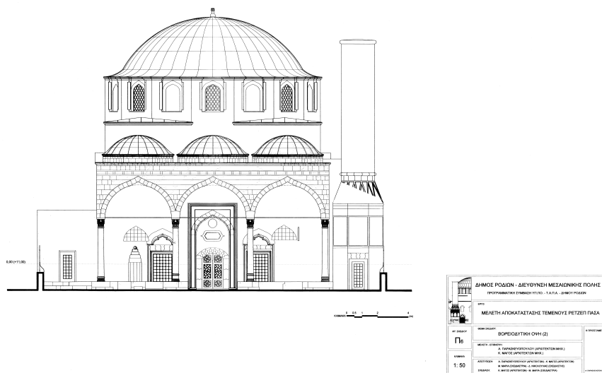
Εικ.: Βορειοδυτική όψη Τεμένους Ρετζέπ Πασά
