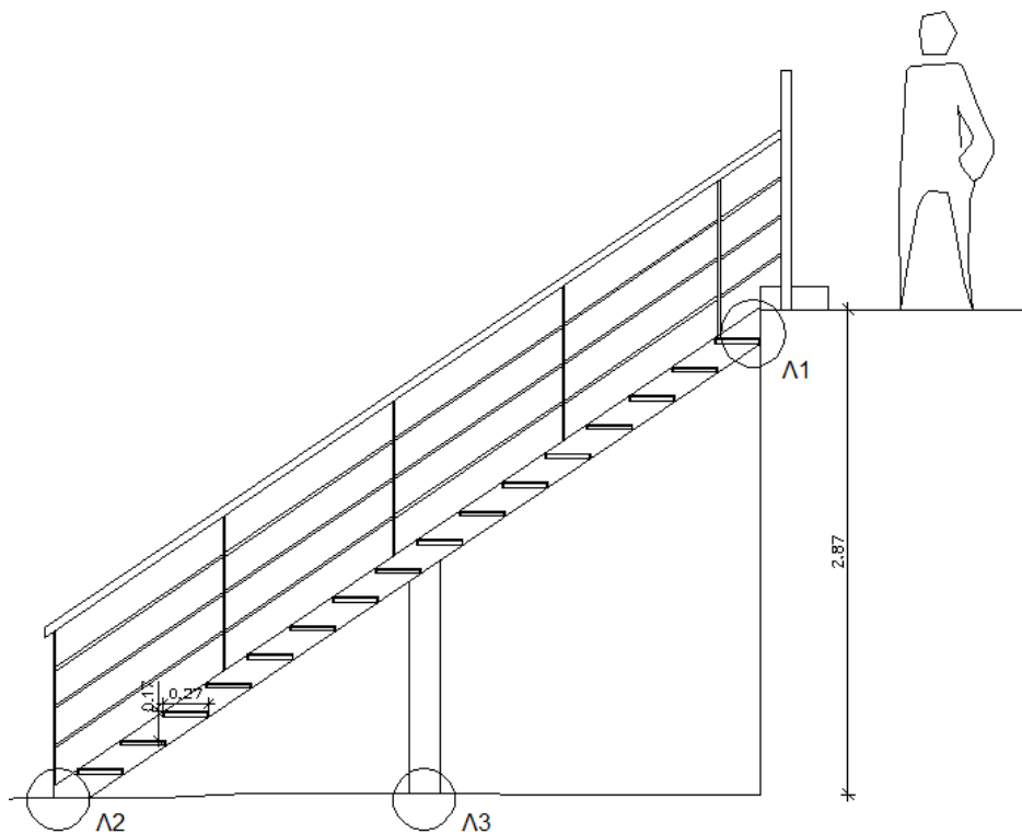
ΤΟΜΗ ΜΕΤΑΛΛΙΚΗΣ ΚΛΙΜΑΚΑΣ
