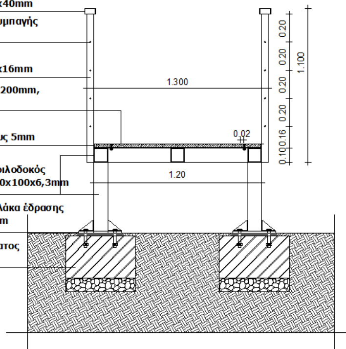
ΕΓΚΑΡΣΙΑ ΤΟΜΗ ΜΕΤΑΛΛΙΚΗΣ ΔΙΑΔΡΟΜΗΣ
