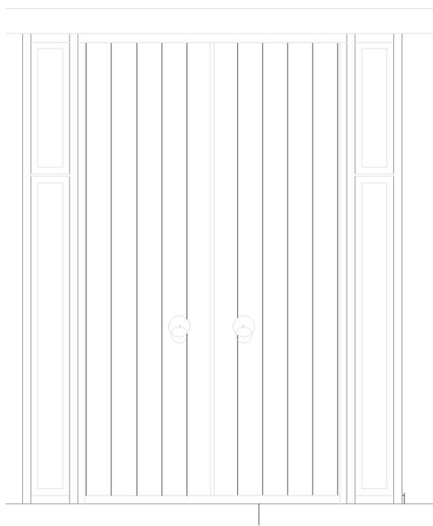
Σχέδιο 2 : Όψη της κεντρικής θύρας διαστάσεων 1,60x2,80 μ., με τα δύο (2) σταθερά υαλοστάσια 0,33x2,80 μ.,
