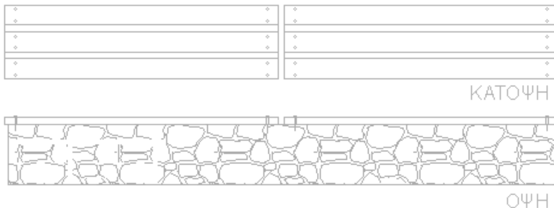
Σχέδιο 10: Ξύλινο παγκάκι - κάτοψη και όψη
