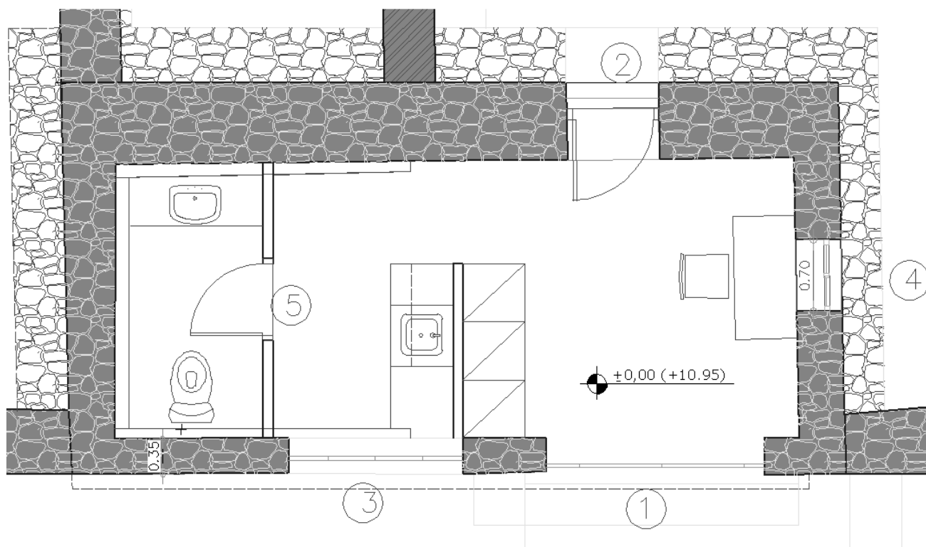
Σχέδιο 1: Κάτοψη ισογείου κτιρίου στην Ρωμαϊκή Έπαυλη, όπου διακρίνονται τα κουφώματα.
