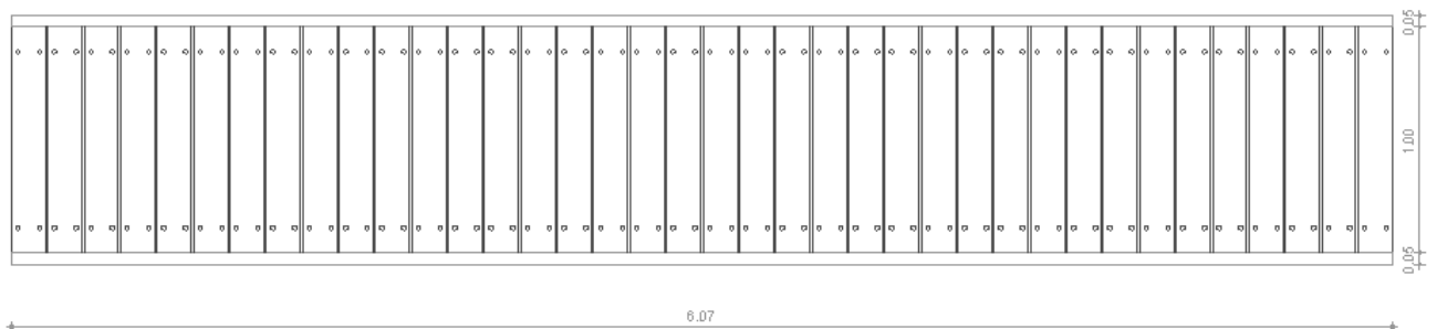
Σχέδιο 18: Κάτοψη ξύλινης διαδρομής
