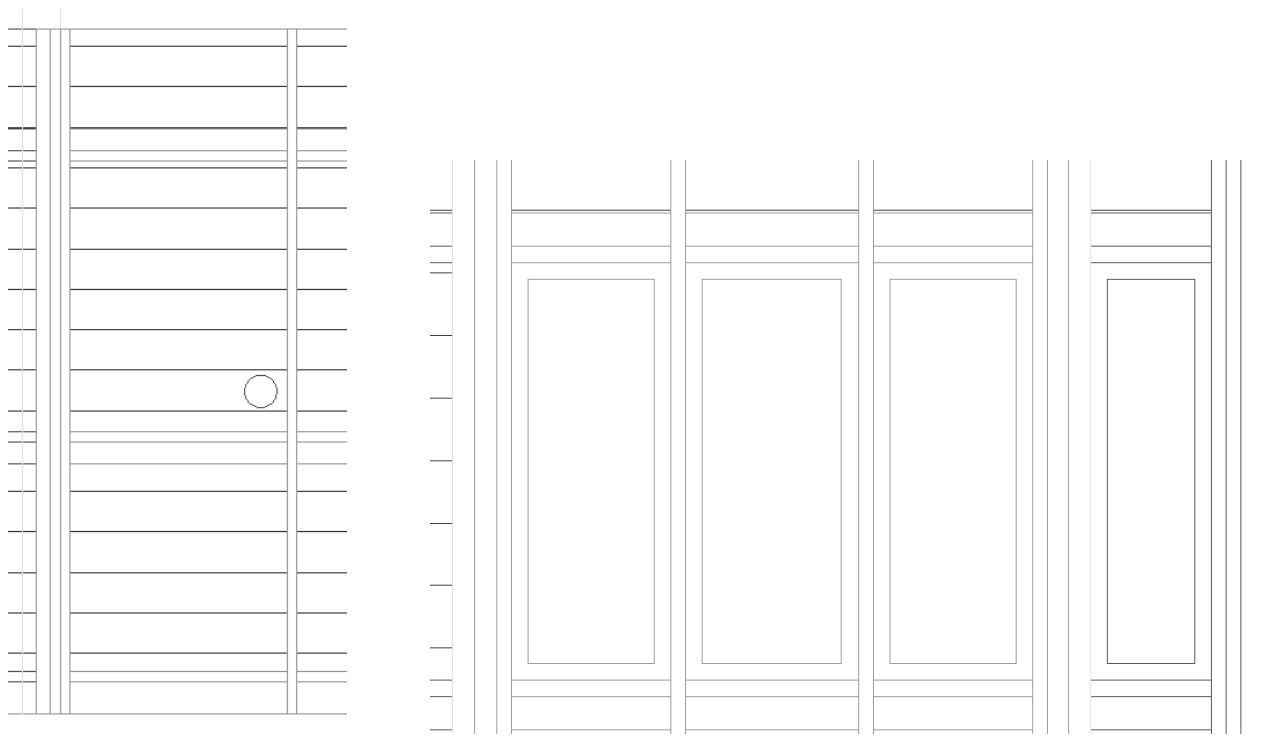
Σχέδιο 12:Εξωτερικά κουφώματα ξύλινου φυλακίου.
