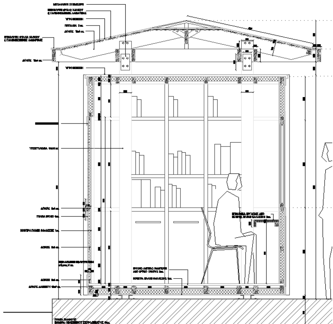
Σχέδιο 14: Τομή ξύλινου φυλακίου
