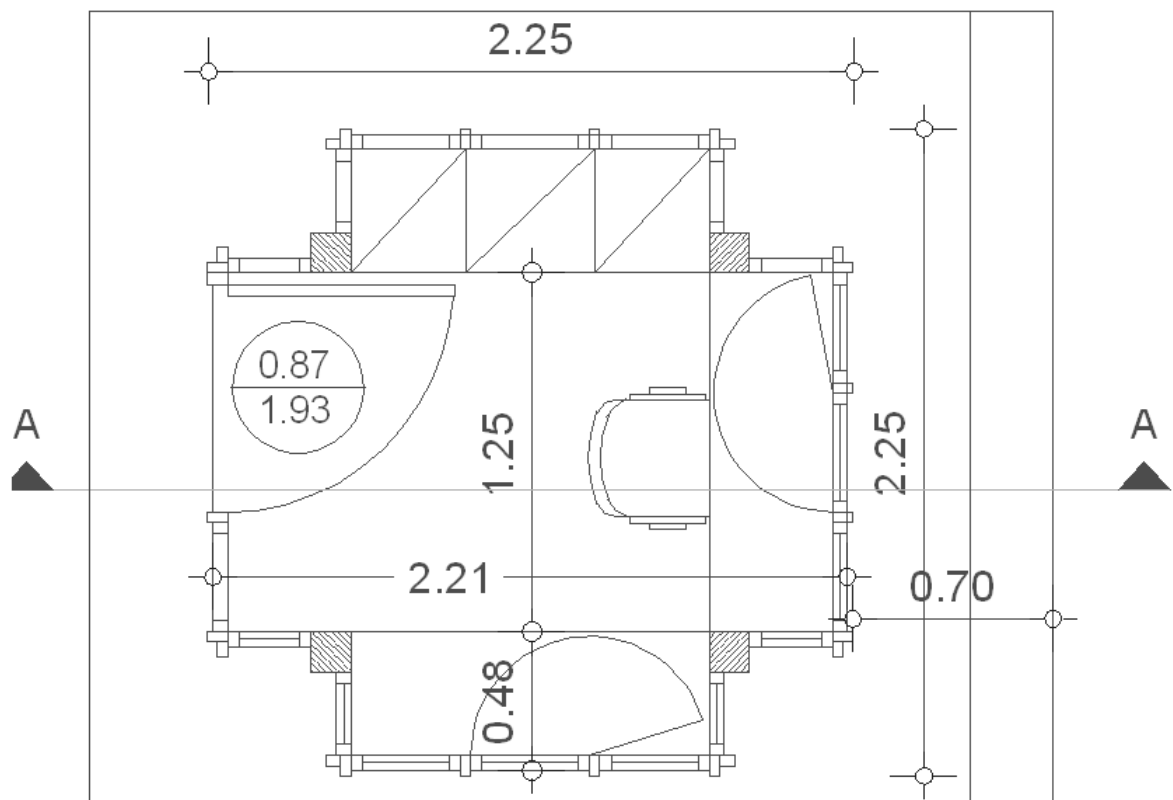
Σχέδιο 11:Κάτοψη ξύλινου φυλακίου.
