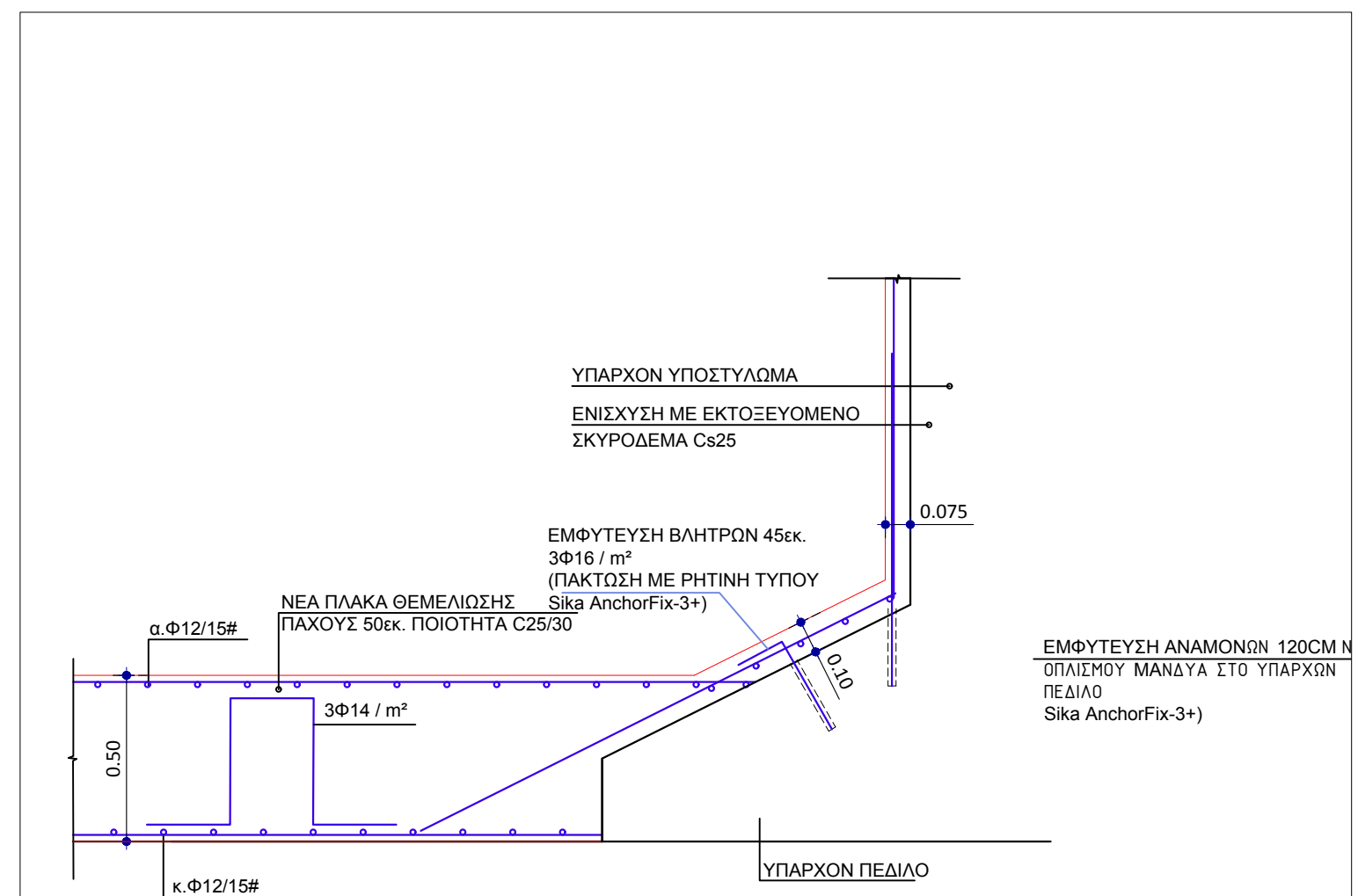
ΤΥΠΙΚΗ ΛΕΠΤΟΜΕΡΕΙΑ ΕΝΙΣΧΥΣΗΣ ΘΕΜΕΛΙΩΣΗΣ ΚΛΙΜΑΚΑ 1:20
