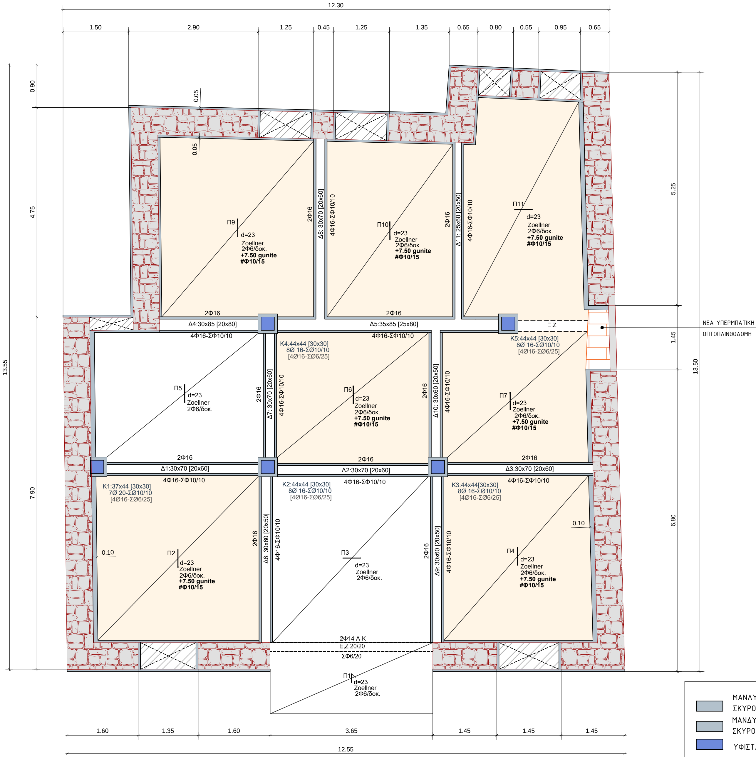
ΞΥΛΟΥΤΥΠΟΣ ΟΡΟΦΗΣ Α' ΟΡΟΦΟΥ-ΕΠΕΜΒΑΣΕΙΣ ΚΛΙΜΑΚΑ 1:50
