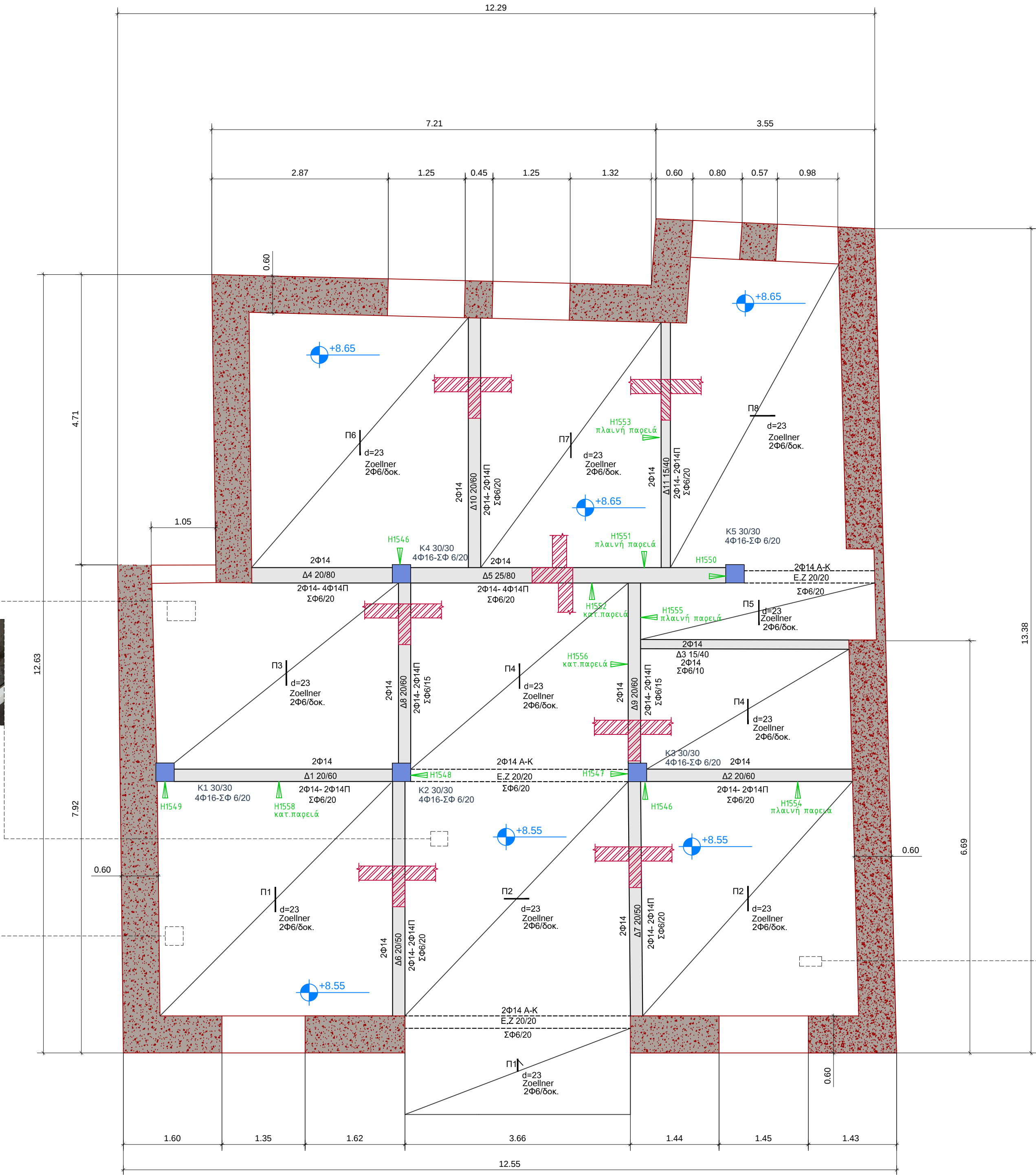
ΞΥΛΟΤΥΠΟΣ ΟΡΟΦΗΣ Α' ΟΡΟΦΟΥ-ΑΠΟΤΥΠΩΣΗ ΚΛΙΜΑΚΑ 1:50
