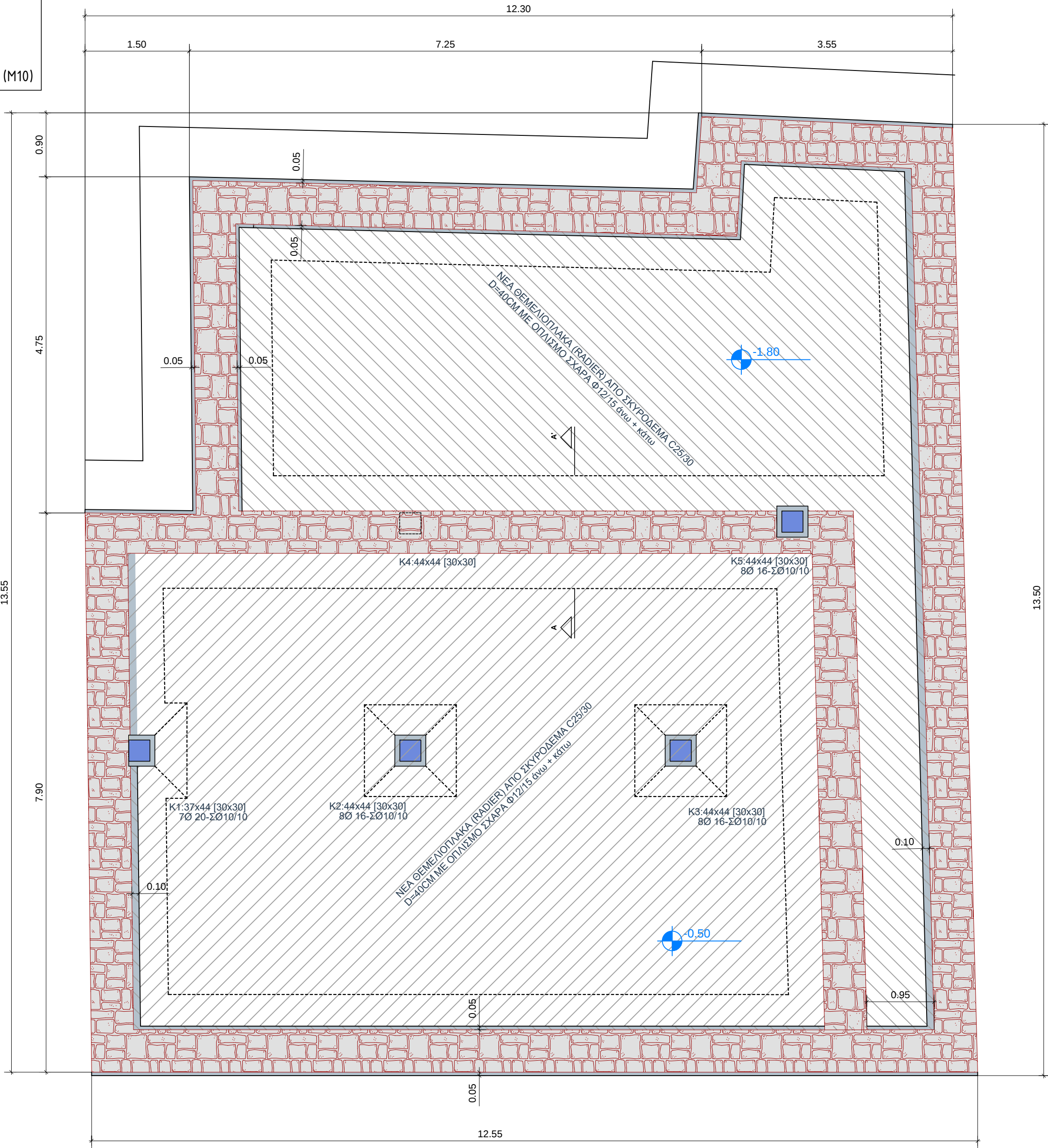
ΞΥΛΟΤΥΠΟΣ ΘΕΜΕΛΙΩΣΗΣ-ΕΠΕΜΒΑΣΕΙΣ ΚΛΙΜΑΚΑ 1:50
