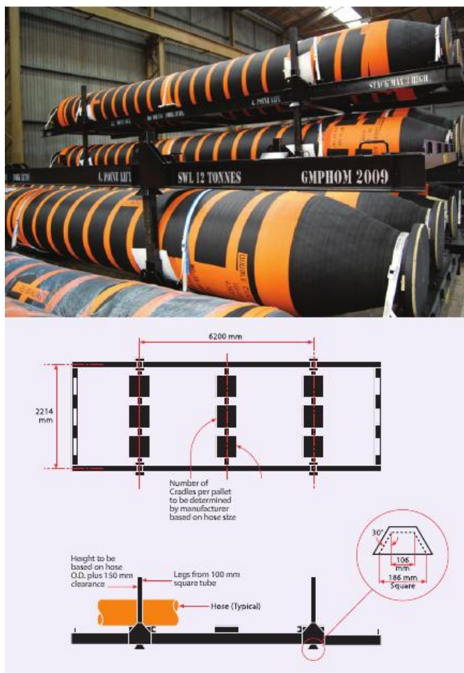
Εικόνα 3: Συσκευασία των υποβρύχιων αγωγών με μεταλλικές εσχάρες.
