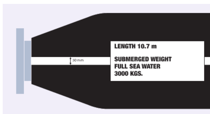
Εικόνα 2: Προβλεπόμενη σήμανση των υποθαλάσσιων αγωγών
