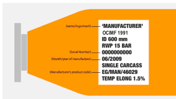
Εικόνα 1: Προβλεπόμενη σήμανση των υποθαλάσσιων αγωγών
