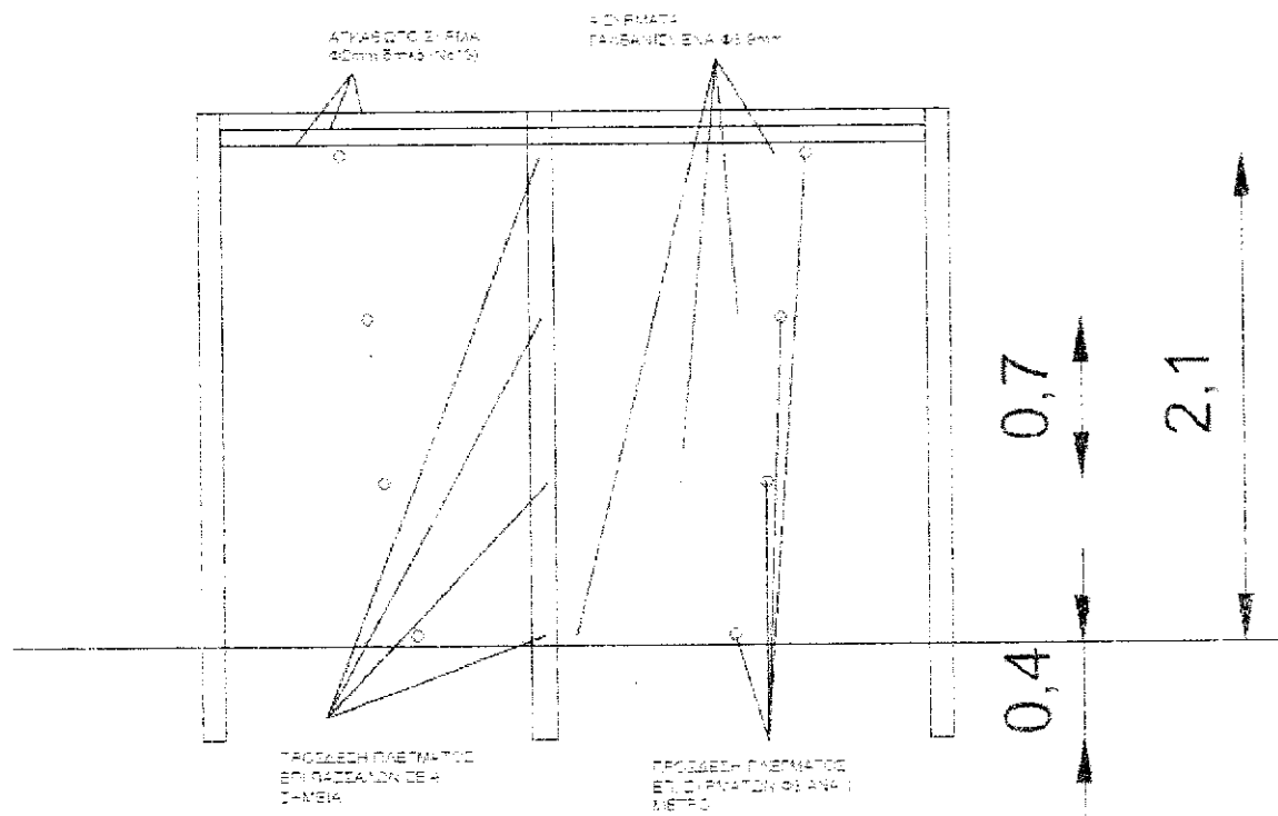
Σχέδιο 1: Όψη περιφράξης.
