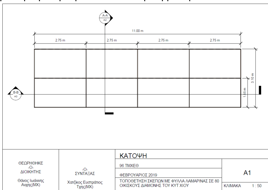
Σχήμα 1: Κάτοψη μεταλλικής σκεπής
