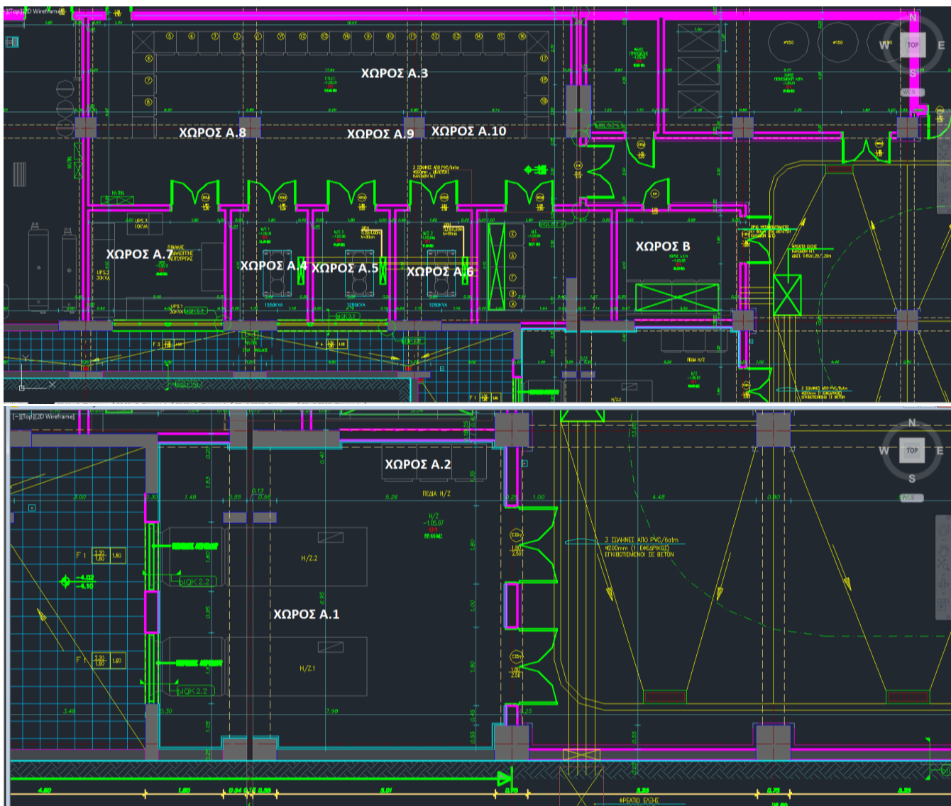
Εικόνα 2. Χώροι επεμβάσεων (αντικατάστασης – εγκατάστασης συστημάτων αυτόματης κατάσβεσης)
