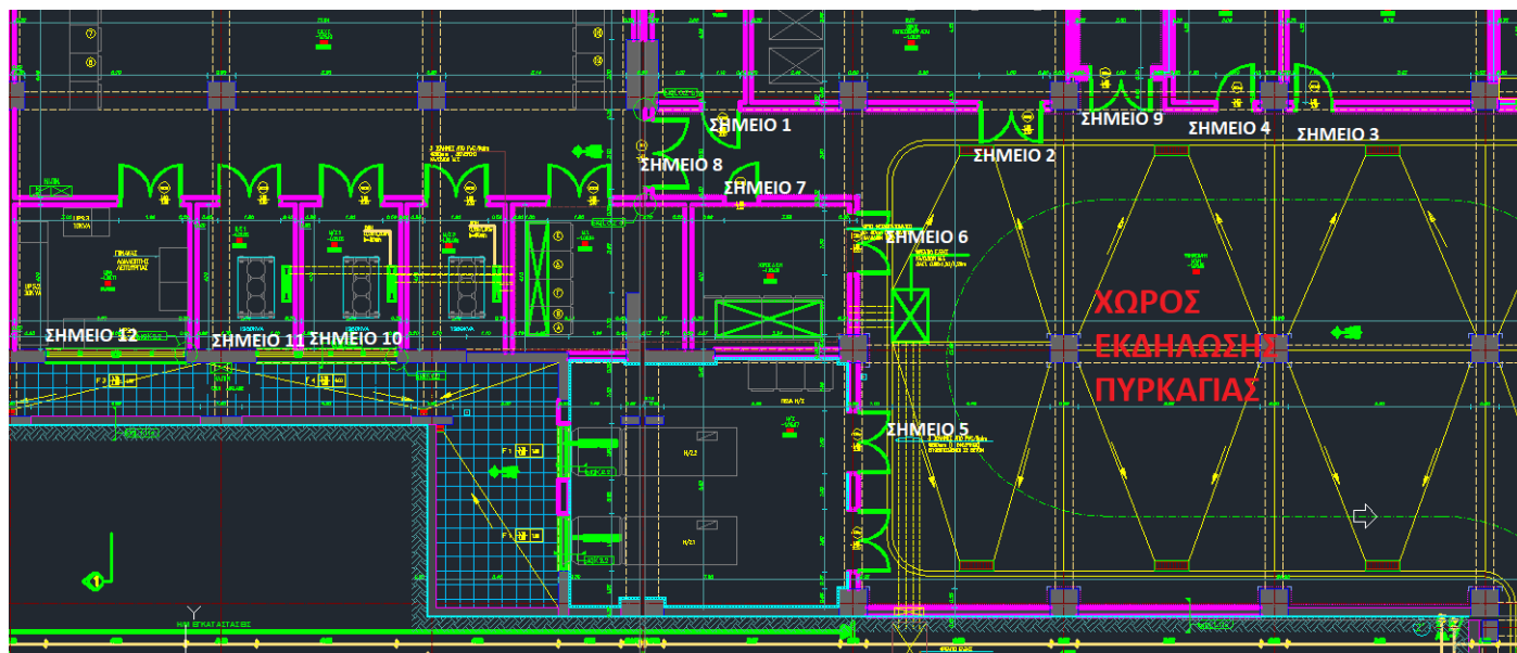
Εικόνα 3. Κάτοψη υπογείου – Σημεία αντικατάστασης θυρών και εγκατάστασης διαφραγμάτων πυρασφάλειας
