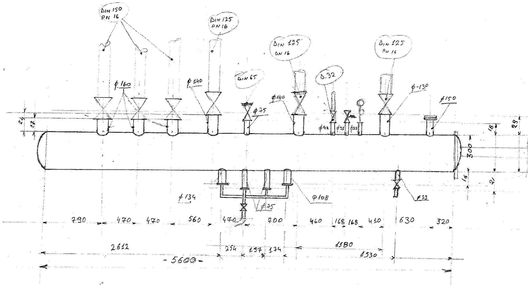
Εικόνα 1. Σκαρίφημα υφιστάμενου ατμοδιανομέα προς αντικατάσταση.
